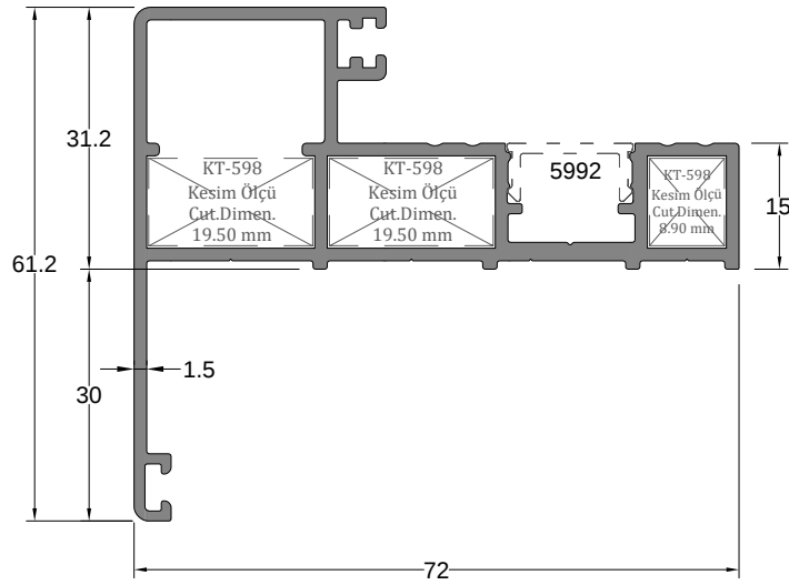
Pervazlı Kasa Profili FRAME PROFILE
