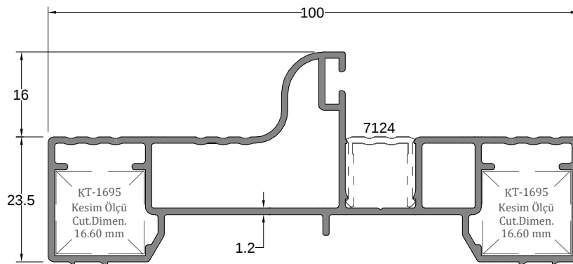
Kapı Kasası Profili DOOR FRAME PROFILE
