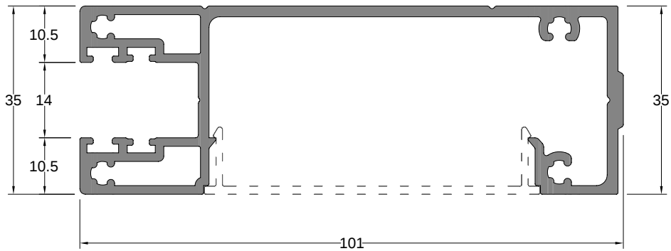
Kablo Kanallı Düşey Kayıt Profili CABLE GROOVE VERTICAL MULLION PROFILE
