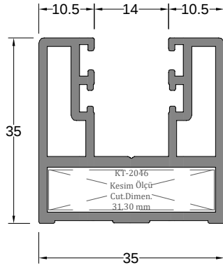
Üst-Yan Kasa Profili TOP-SIDE FRAME PROFILE
