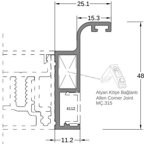
Pervazlı Kasa Profili SILL FRAME PROFILE
