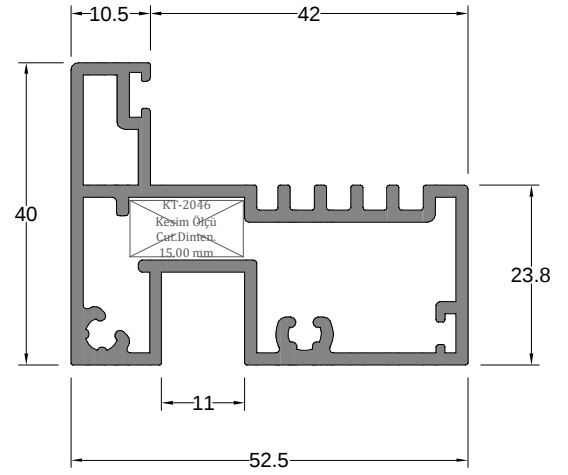
Kapı Kasası Profili DOOR PROFILE
